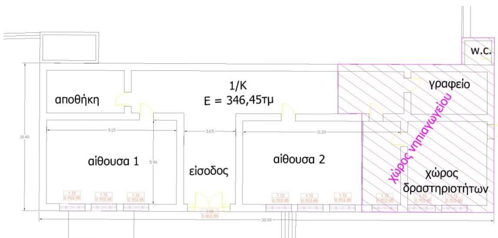
Σχήμα 1. Υφιστάμενη διαρρύθμιση κτιρίου
