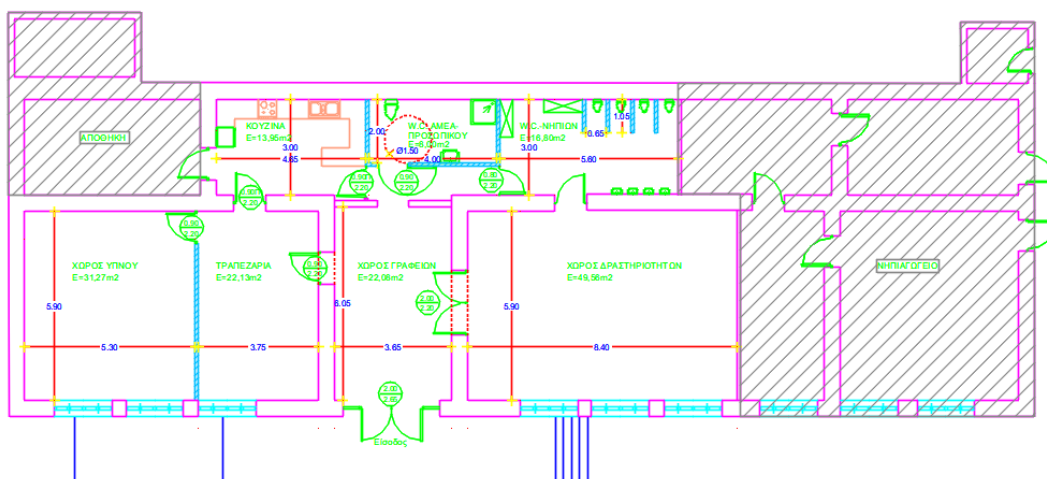
Σχήμα 2. Πρόταση διαρρύθμισης κτιρίου για τη στέγαση του παιδικού σταθμού
